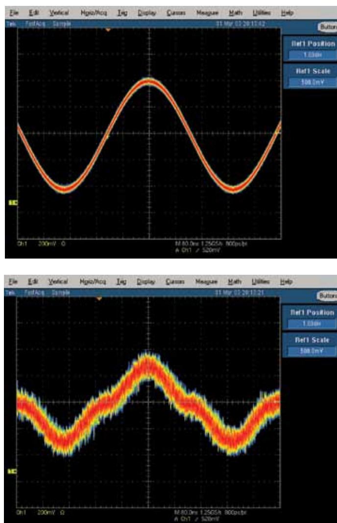
Рис. 2. Идеальный сигнал (вверху) и реальный сигнал (внизу). Универсальный генератор сигналов может вносить контролируемые искажения для тестирования и измерения параметров устройств в предельных режимах работы.
